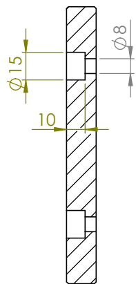
剖面圖 A-A
