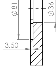
剖面圖 B-B
