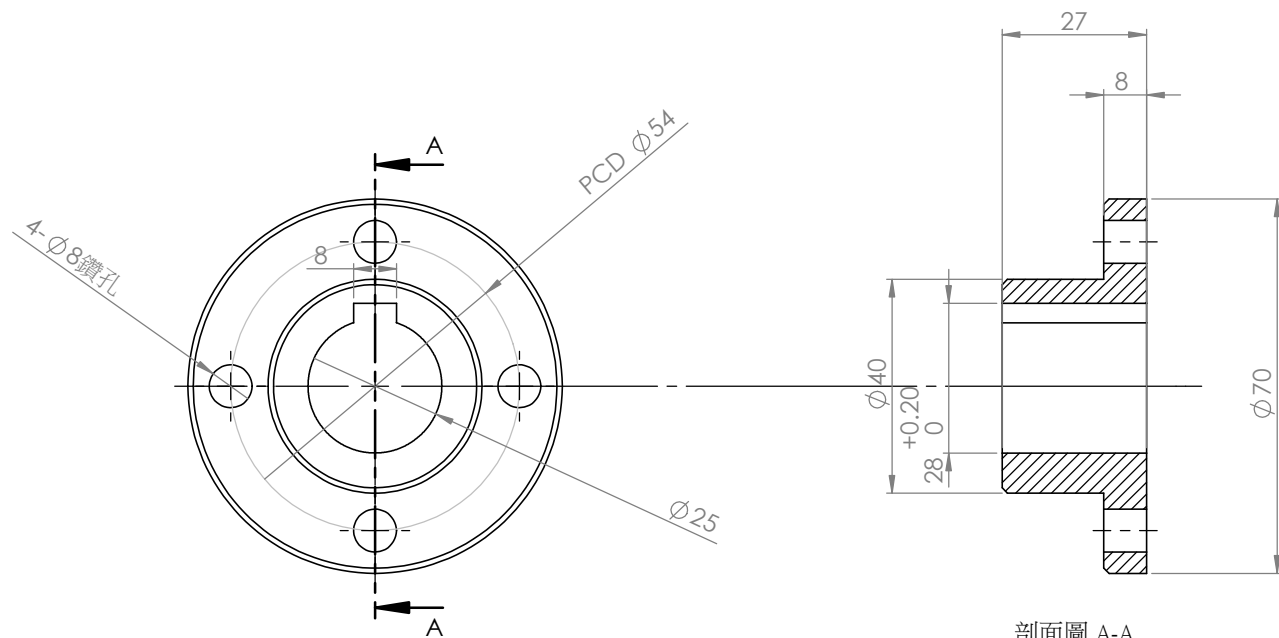
剖面圖 A-A
