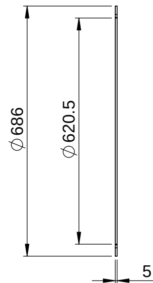
剖面圖 A-A
