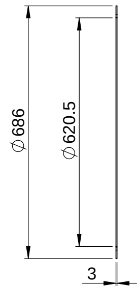
剖面圖 A-A
