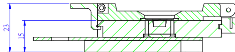
剖面 A-A
