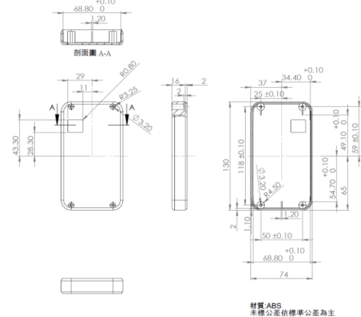
32陣列後殼
