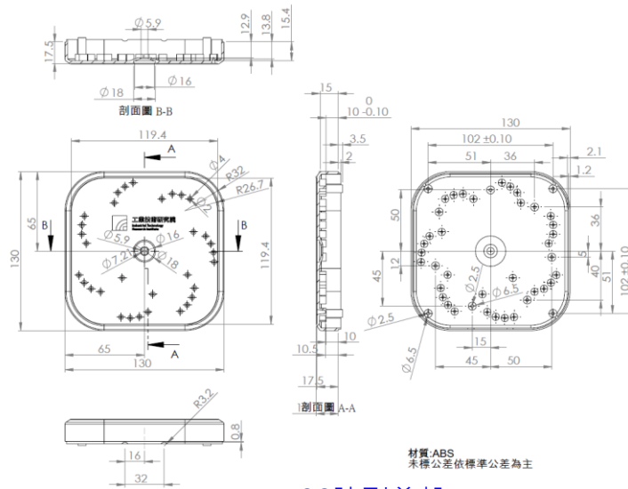
32陣列前殼
