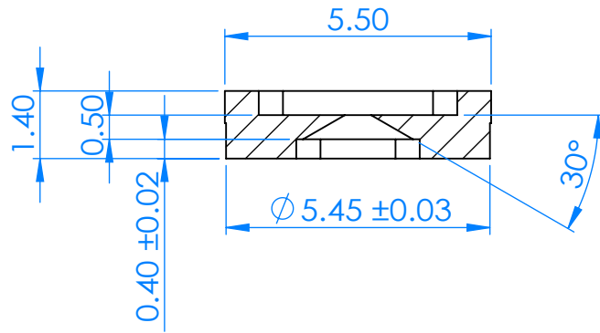
剖面圖 A-A 縮放 7:1
