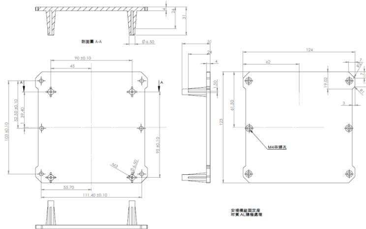
安堤模組固定座
