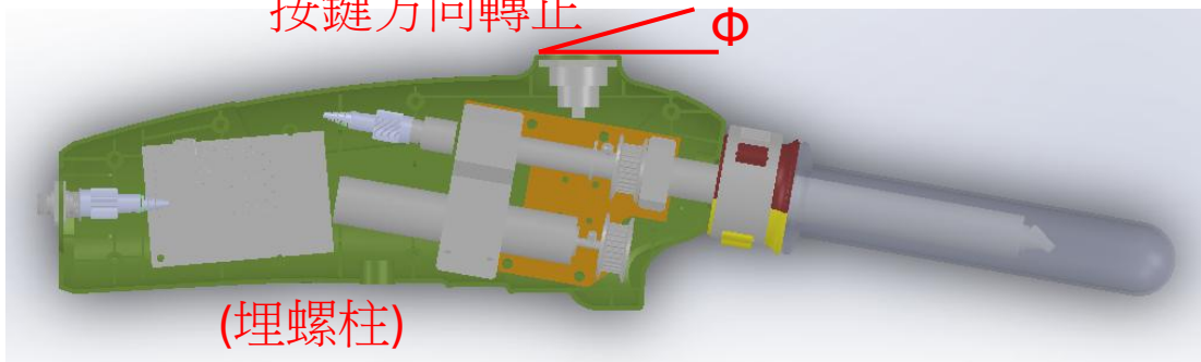
人因探頭三視圖
