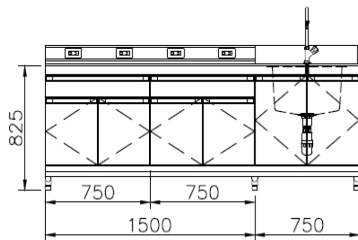
立面圖
