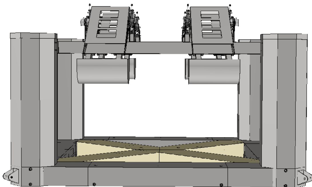
圖 2、浮台平台示意圖(尺寸僅供參考，實際尺寸於訂單成立後提供)
