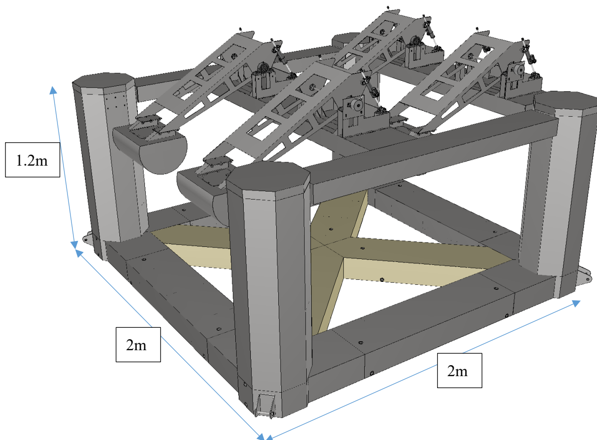
圖 1、浮台平台示意圖(尺寸僅供參考，實際尺寸於訂單成立後提供)
