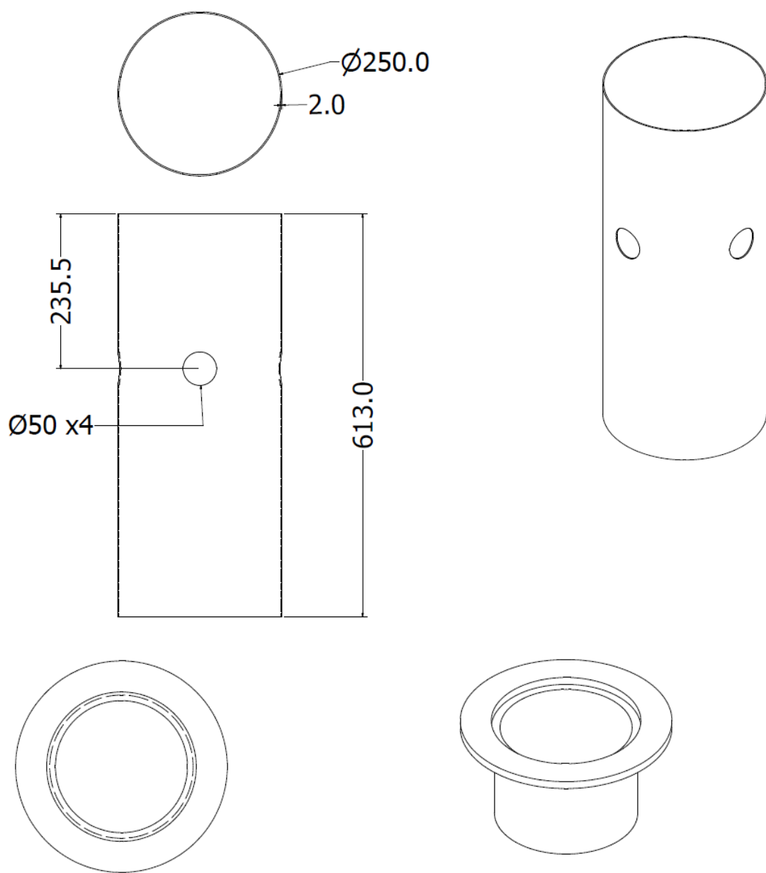
SUS316 NW50長頸接頭
