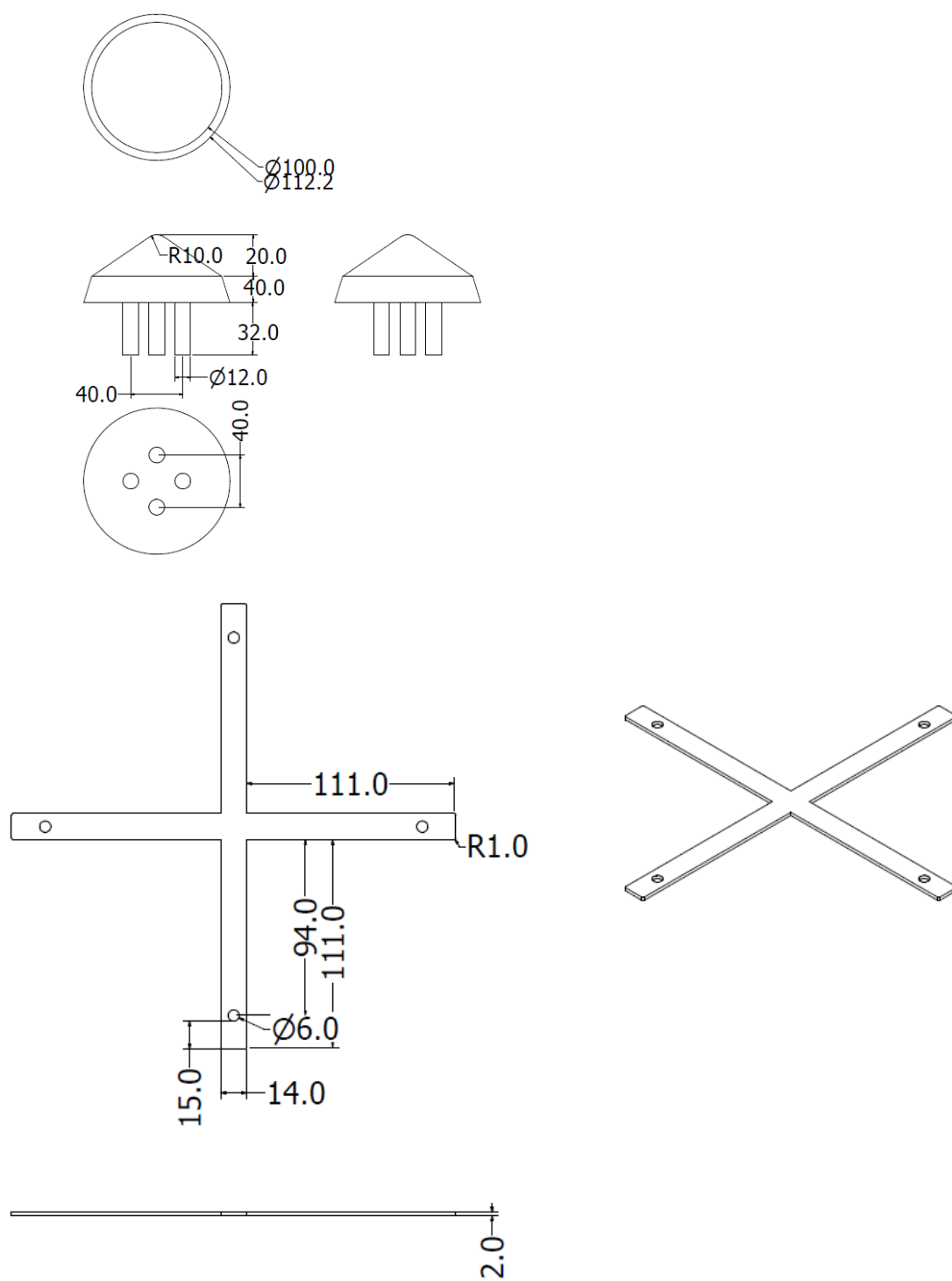
8. 內襯管組合 x1
