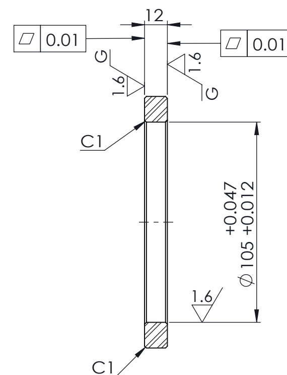
剖面圖 A-A
