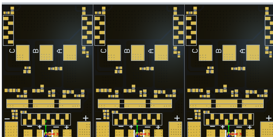
圖二. 電路板 B
