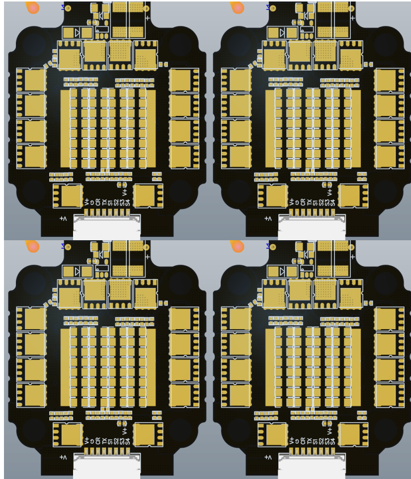
圖一. 電路板 A
