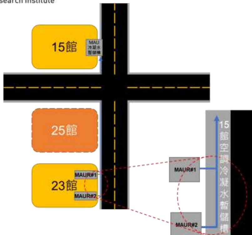
圖 3. 維護完畢管路路線(示意圖)
