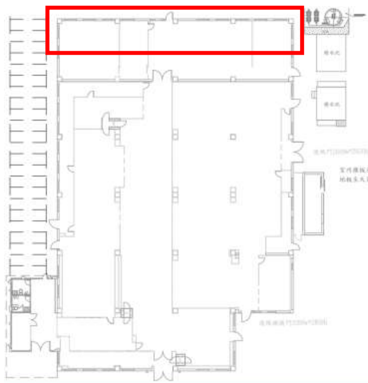
圖 1. 23 館空調冷凝水管路維護
