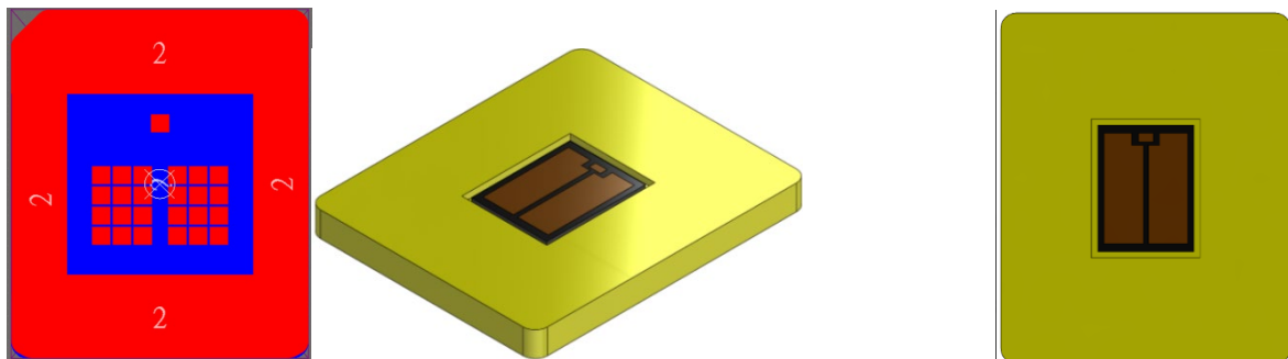
圖3 嵌入式子模組尺寸圖.
