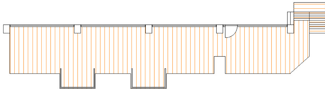
南方松木棧板平台拆除範圍
