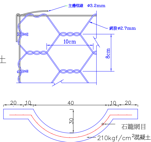
石籠及平台拍漿溝詳圖 單位：cm
