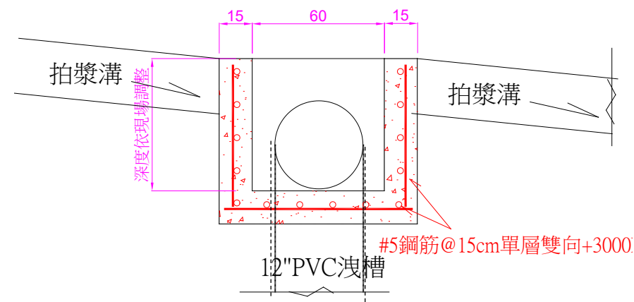
新設集水井詳圖 單位：cm
