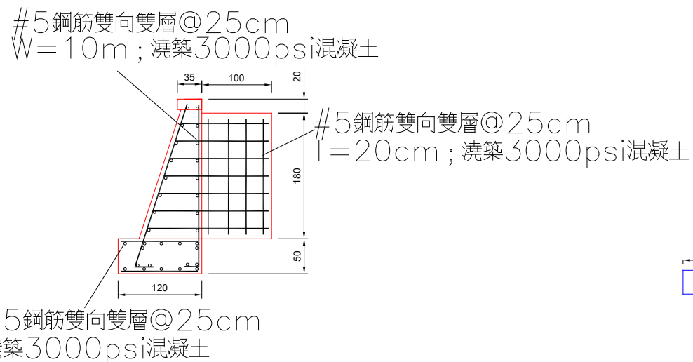
擋土牆配筋詳圖 單位：cm
