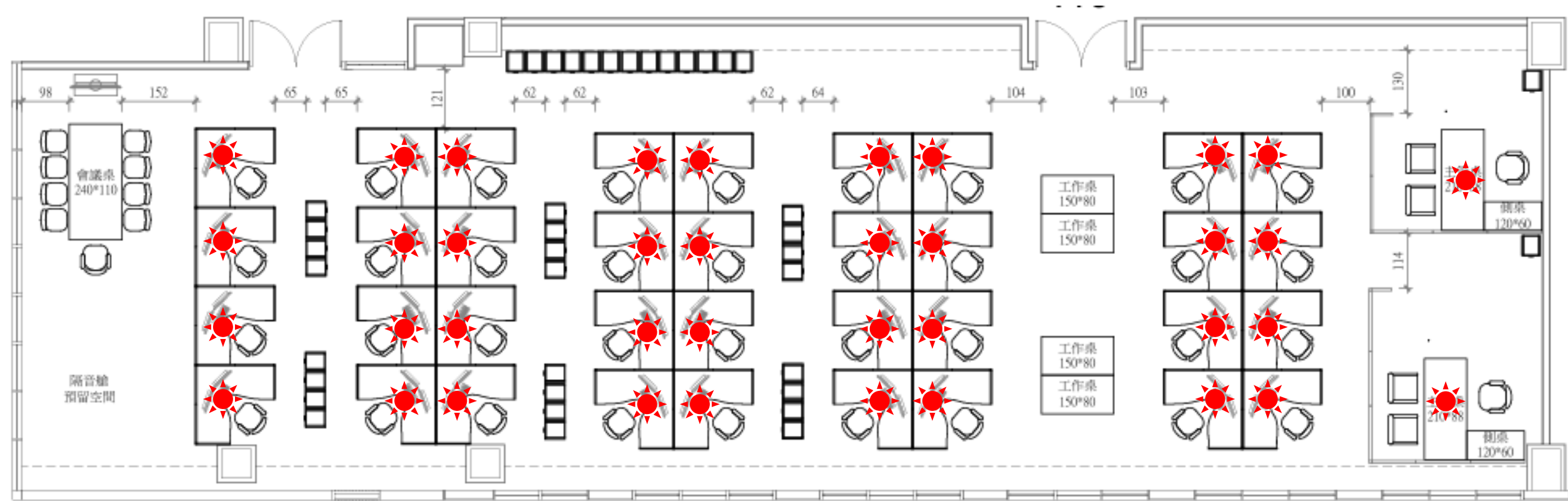
B419增設光源配置規劃圖
