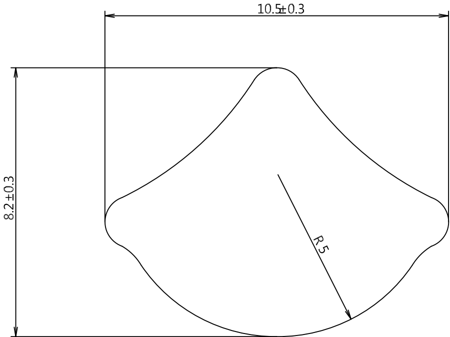
截面詳圖
