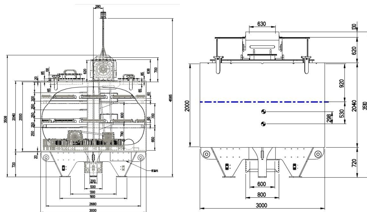
圖 1、波浪發電機組外型尺寸規格
