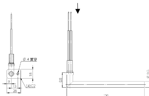
6.加熱棒 10-130L 直角 220V200W
