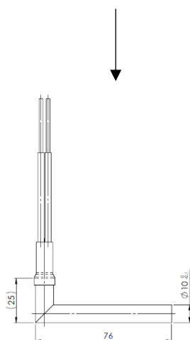
4.加熱棒 10-110L 直角 220V150W
