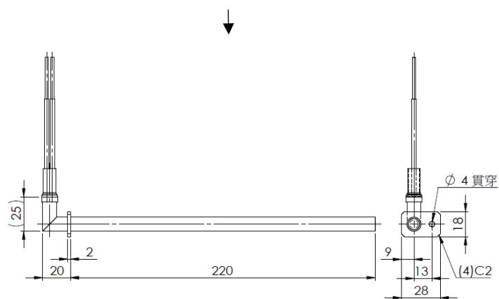
9.加熱棒 10-220L 直角 220V300W
