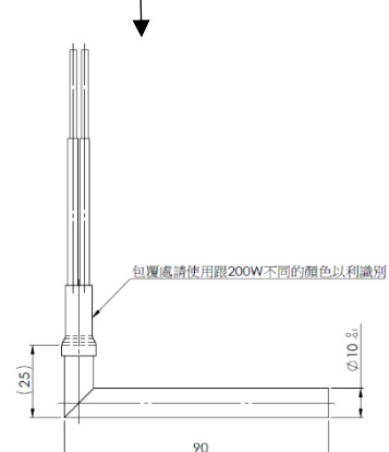
3.加熱棒 10-90L 直角 220V150W
