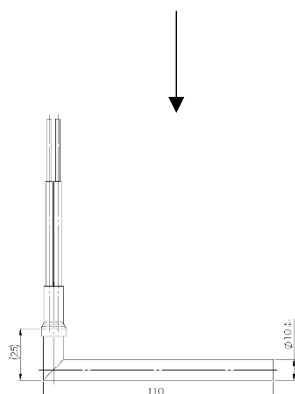
4.加熱棒 10-110L 直角 220V150W
