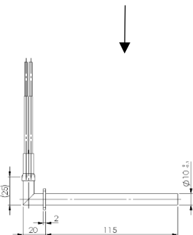
5.加熱棒 10-115L 直角 220V200W
